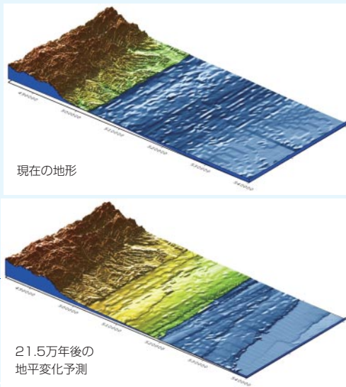
図3 現在の地形と21.5万年後の地平変化予測（海水準：現在比±0m）
